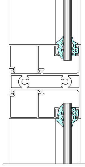
DETAIL 2 ( T-verbinding ) ( travers )
