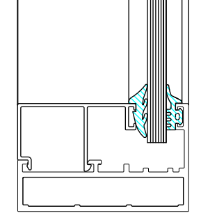
DETAIL 1 ( buitenkader ) ( cadre )
